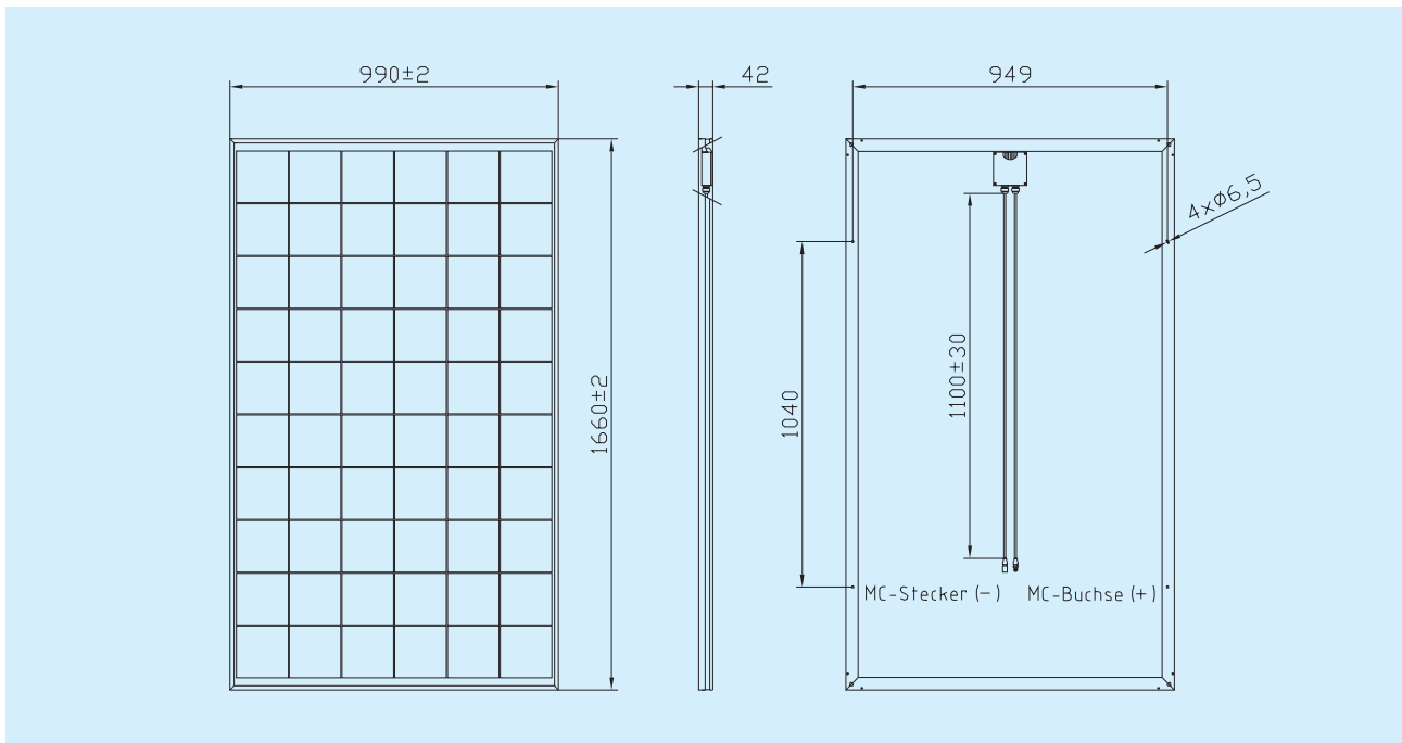
Maßzeichnung IBC-220TS MEGALINE
